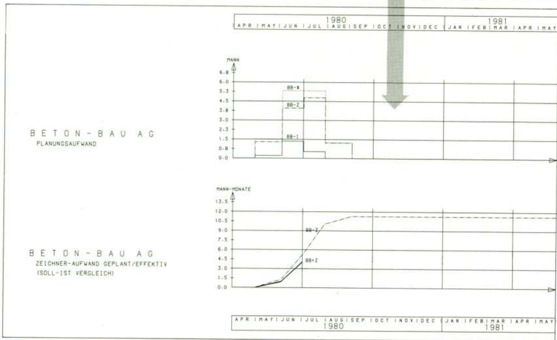
Bild 9. Kombinierte Plot-Darstellung der Termin- und Einsatzmittelplanung: Balkendiagramm, Einsatzmittel-Plan und Einsatzmittel-Verteilkurven
