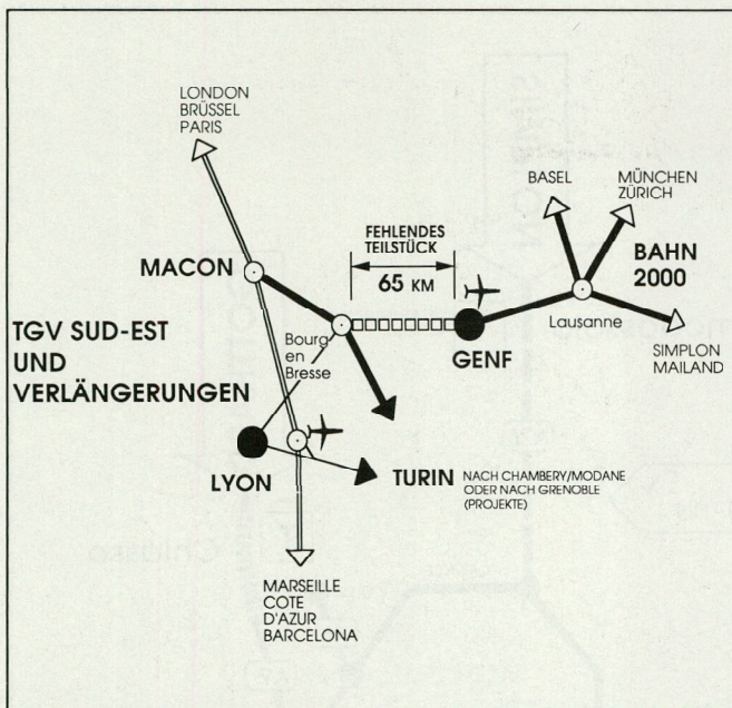
Bild 10 – Genf–Bourg-en-Bresse, ein relativ kurzes fehlendes Teilstück zwischen dem schweizerischen Netz von BAHN 2000 und der TGV-Achse Paris-Südost mit ihren Verlängerungen gegen die Côte d'Azur und Barcelona.
