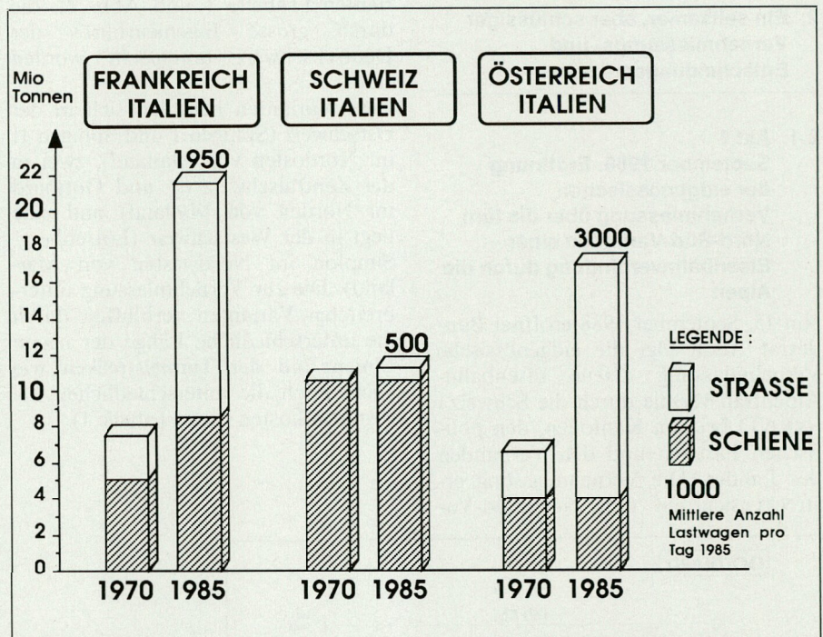
Bild 1 - Entwicklung 1970-1985 des transalpinen Güterverkehrs, welche das phänomenale Wachstum des Schwerverkehrs zeigt. Dieses Wachstum kann nicht unbeschränkt weitergehen, ohne schwerwiegende Probleme der Verstopfung von transalpinen Strassen- und Autobahnachsen und einer in den Alpentälern schwer zu meisternden Umweltbelastung zu schaffen.
