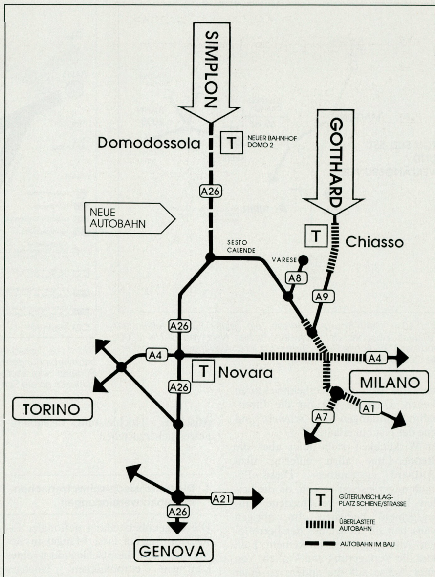
Bild 12 – Anschluss der Eisenbahnachsen des Simplon und des Gotthard an das Autobahnnetz von Norditalien. Die Güter-Umschlagplätze Schiene-Strasse der Gotthard-Achse liegen am Rande des überlasteten Autobahnnetzes der Region Mailand. Dank der im Bau befindlichen Autobahn A26 wird die Simplon-Achse von einer Verteilung des Verkehrs gegen die drei Pole Mailand, Genua und Turin unter Vermeidung der «Passage obligé» von Mailand profitieren.
