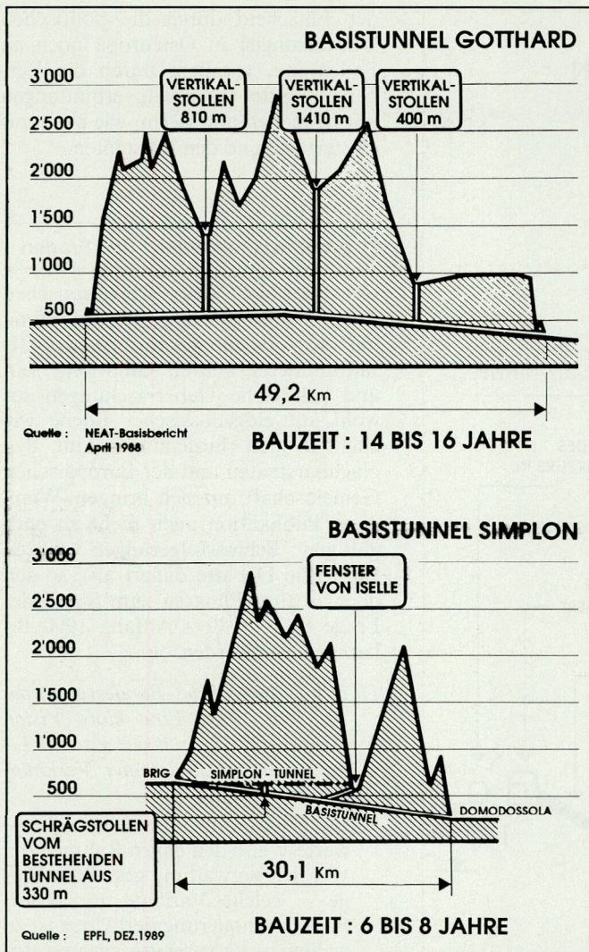
Bild 13 – Merkmale und Zwänge für den Durchstich der Basistunnel am Gotthard und am Simplon. Indem er sich im bestehenden Tunnel abstützt, kann der Simplon-Basistunnel ohne die gigantischen Vertikalstollen gebaut werden, die für den Durchstich des Gotthard-Basistunnels notwendig sind. Sowohl Kosten wie auch Bauzeit wären für den Simplon-Tunnel wesentlich geringer.
