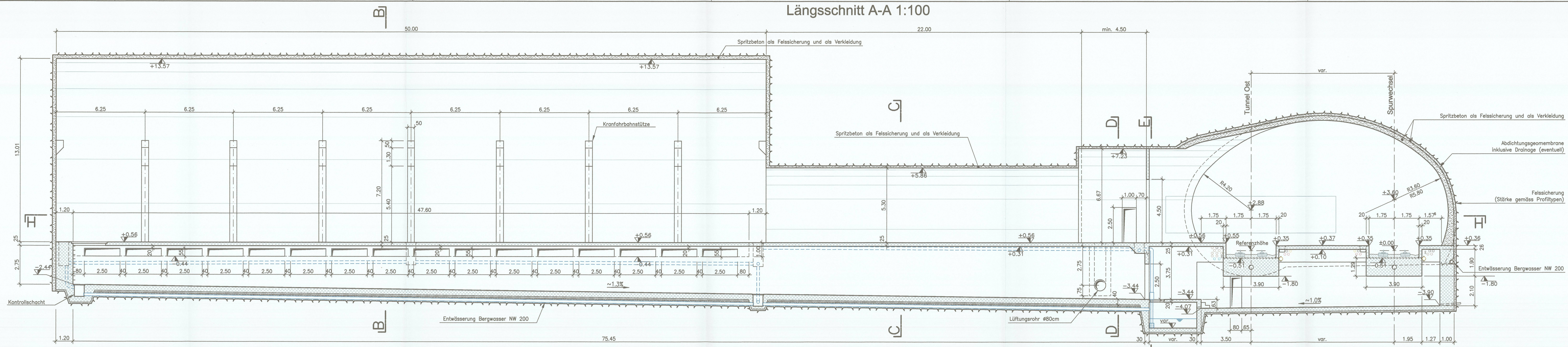
Längsschnitt A-A 1:100
